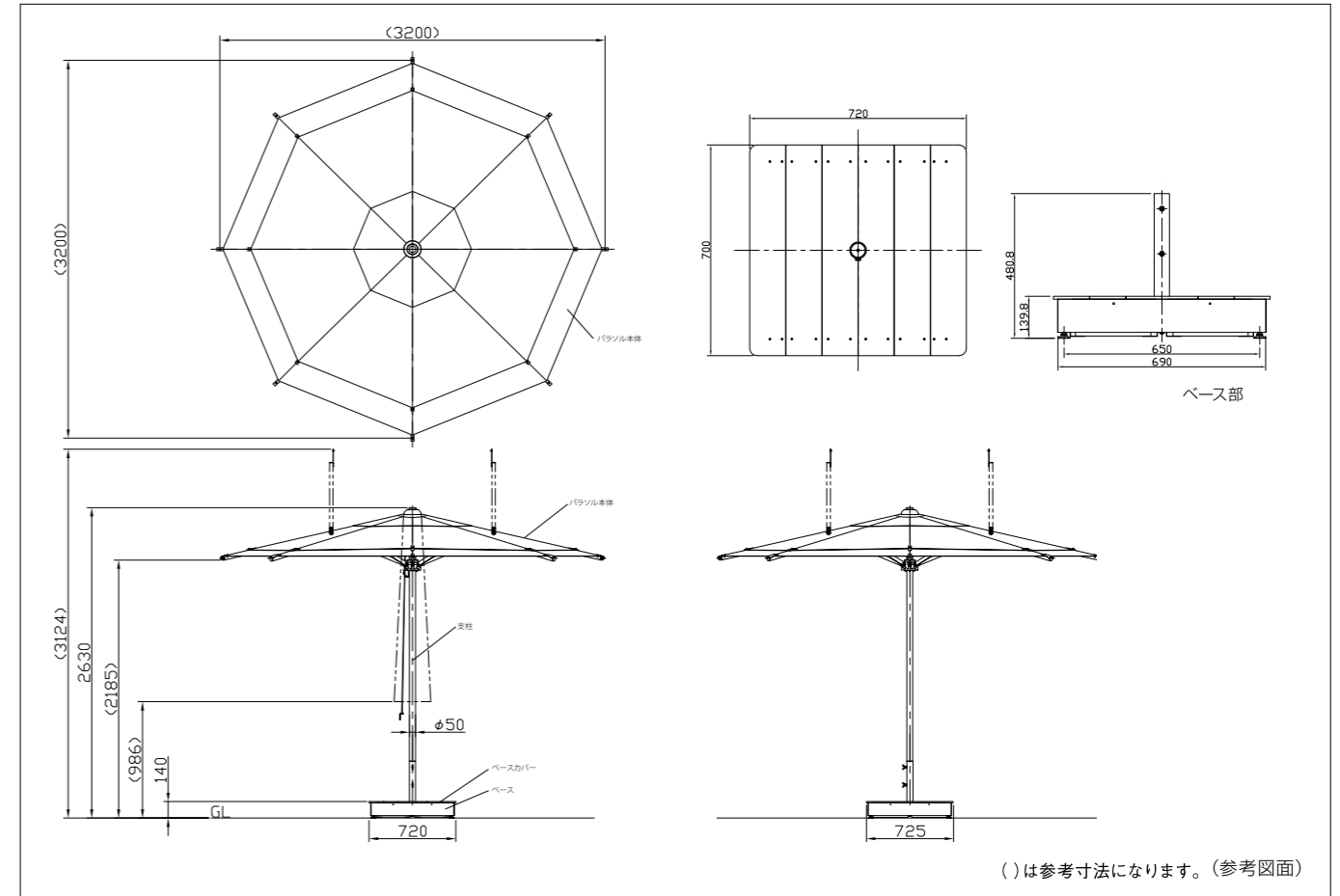
ステラ CP (センターポール) 基本寸法図
